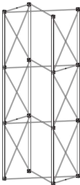
Položka č.: 2.50.13001 Váha: 5,3 kg Materiál: slitina hliníku, eloxovaná
