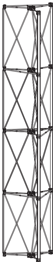
Položka č.: 2.50.14002 Váha: 6,96 kg Materiál: slitina hliníku, eloxovaná
