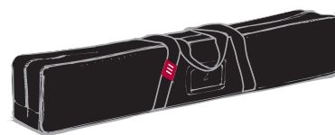
Položka č.: 2.51.07001-01 Váha: 1,86 kg Materiál: nylon, molitan Rozměry: 100 x 12 x 18 cm
