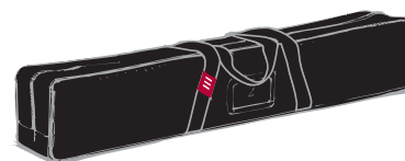
Položka č.: 2.51.07001-01 Váha: 1,86 kg Materiál: nylon, foam filling Rozměry: 100 x 12 x 18 cm
