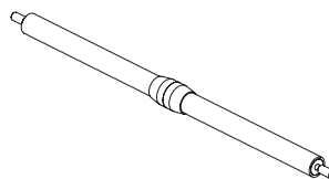
Položka č.: 2.46.09003 Váha: 0,04 kg Materiál: slitina hliníku, eloxovaná plast, magnet
