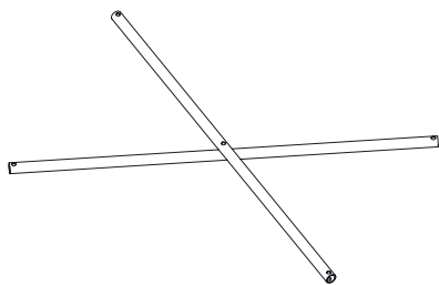
Položka č.: 2.46.09001 Váha: 0,05 kg Materiál: slitina hliníku, eloxovaná
