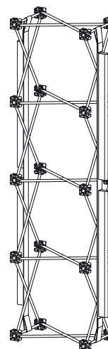
Položka č.: 2.48.06013 2.48.06014 2.48.06015 Váha: 1,2; 2,5; 2,7 kg Materiál: velcro (bílý), plast
