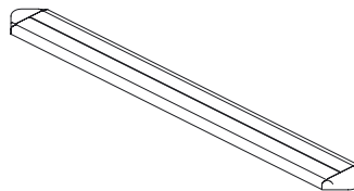
Položka č.: 2.46.01001 Váha: 0,12 kg Materiál: slitina hliníku, eloxovaná magnetická páska
