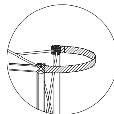
Položka č.: 2.41.01180 Váha: 0,10 kg Materiál: slitina hliníku s magnetickou páskou
