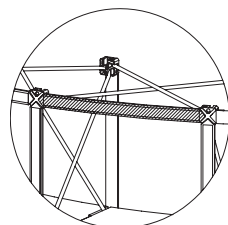
Položka č.: 2.41.01012 Váha: 0,17 kg Materiál: slitina hliníku s magnetickou páskou
